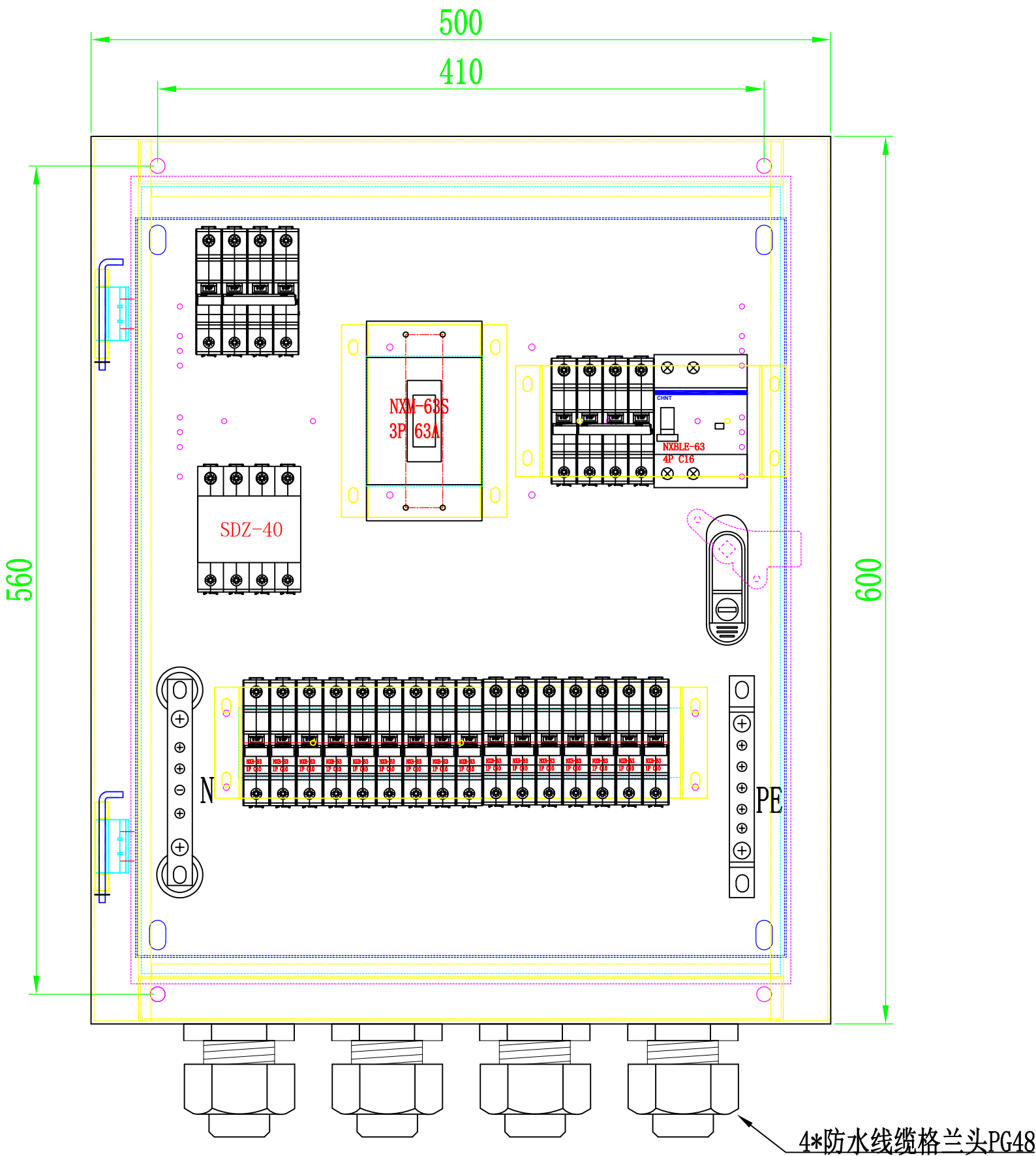
(带元器件)照明箱 500*600(内外门) 配有支架, 断路器, 零排, 地排 防水接头PG48
