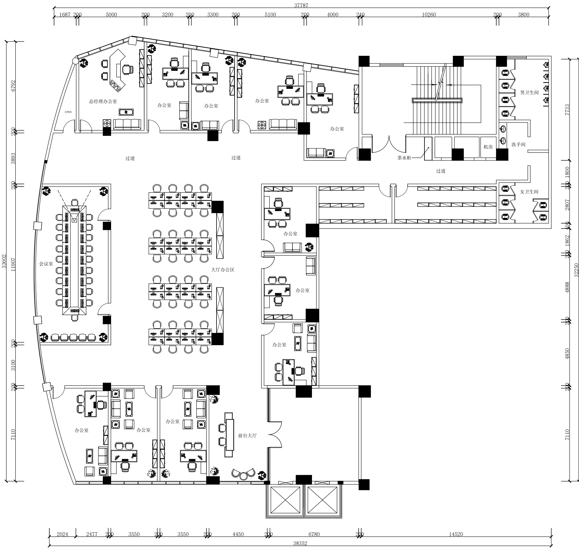
北部湾保险北海分公司平面布置图
