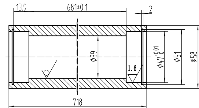
件2: 辊筒
