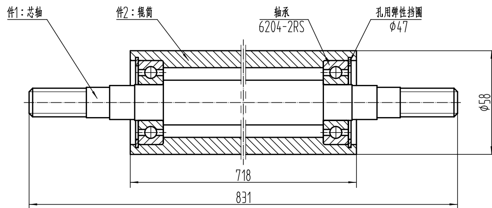
装配图
