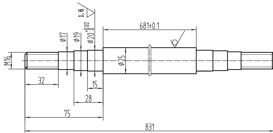
件1: 芯轴
