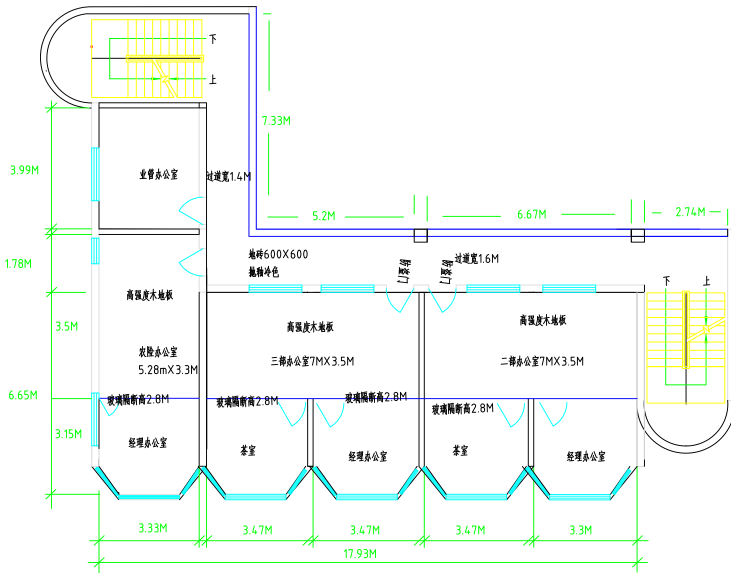
三层平面图
