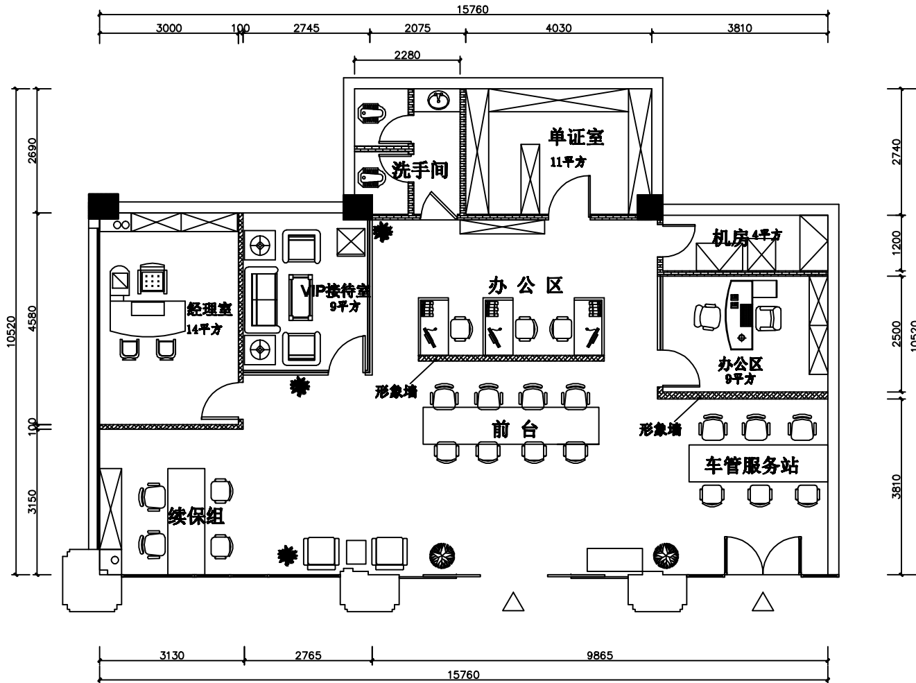
平面布置图1:100
