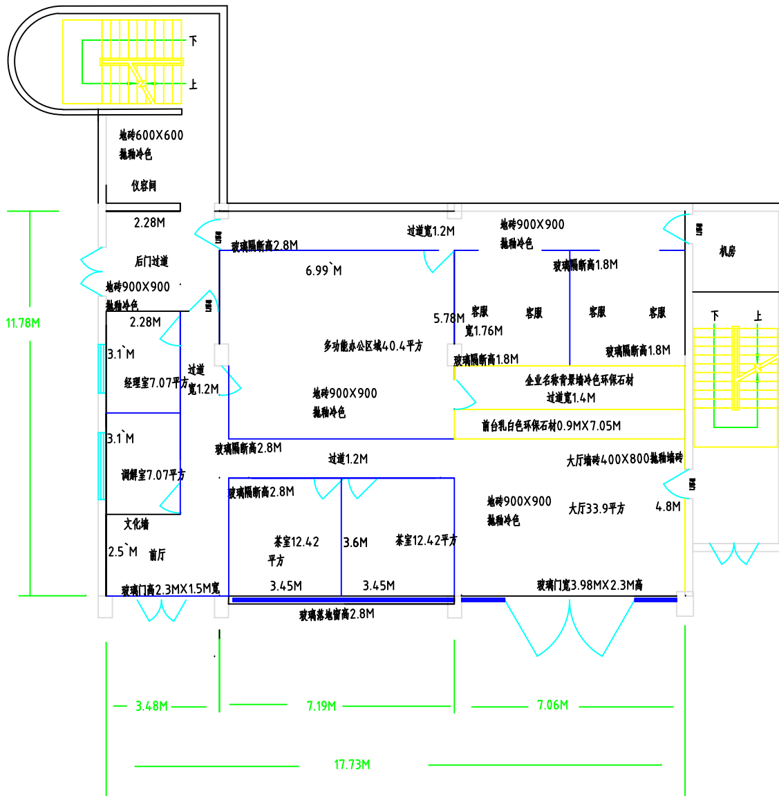
一层大厅平面图
