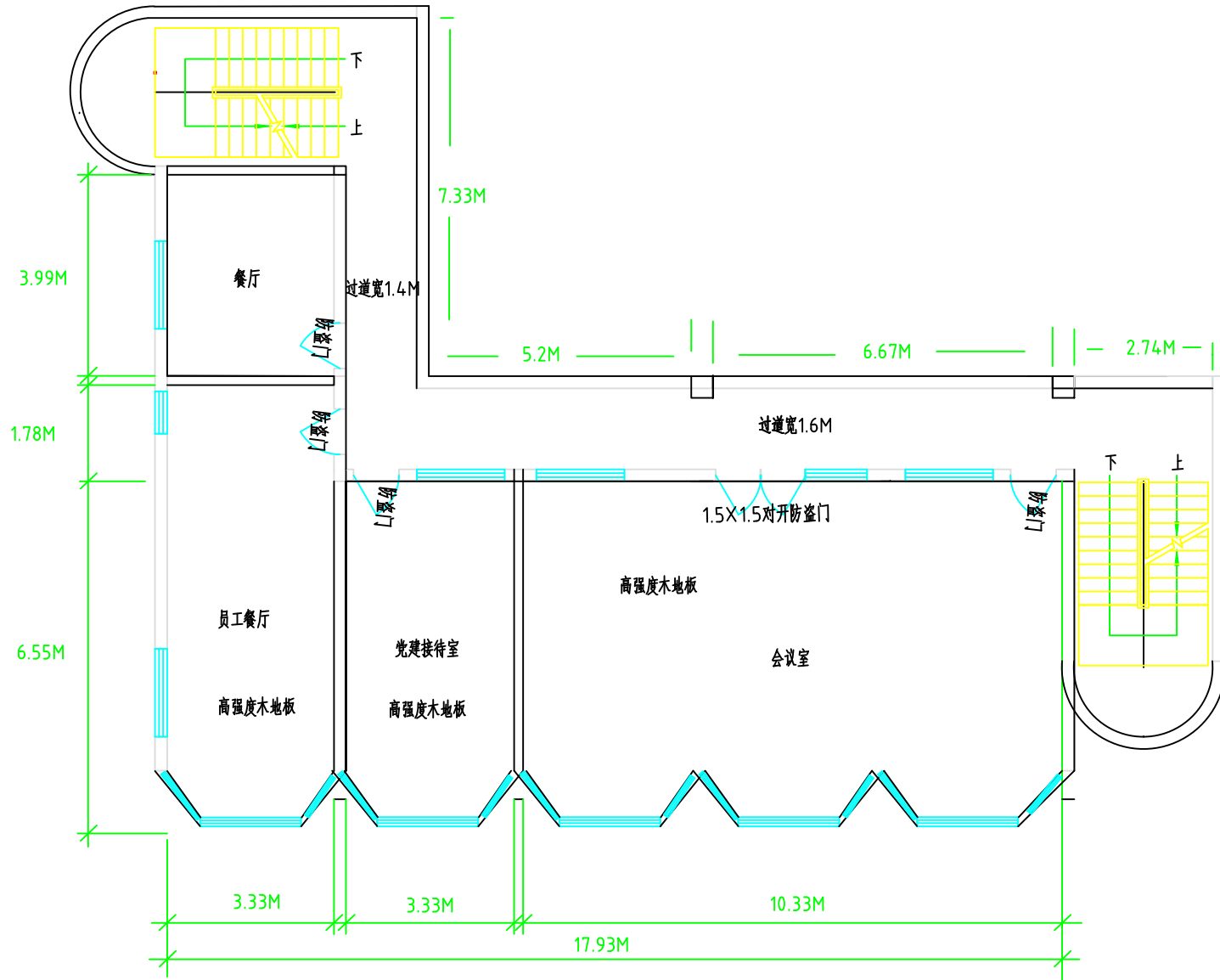
五层平面图
