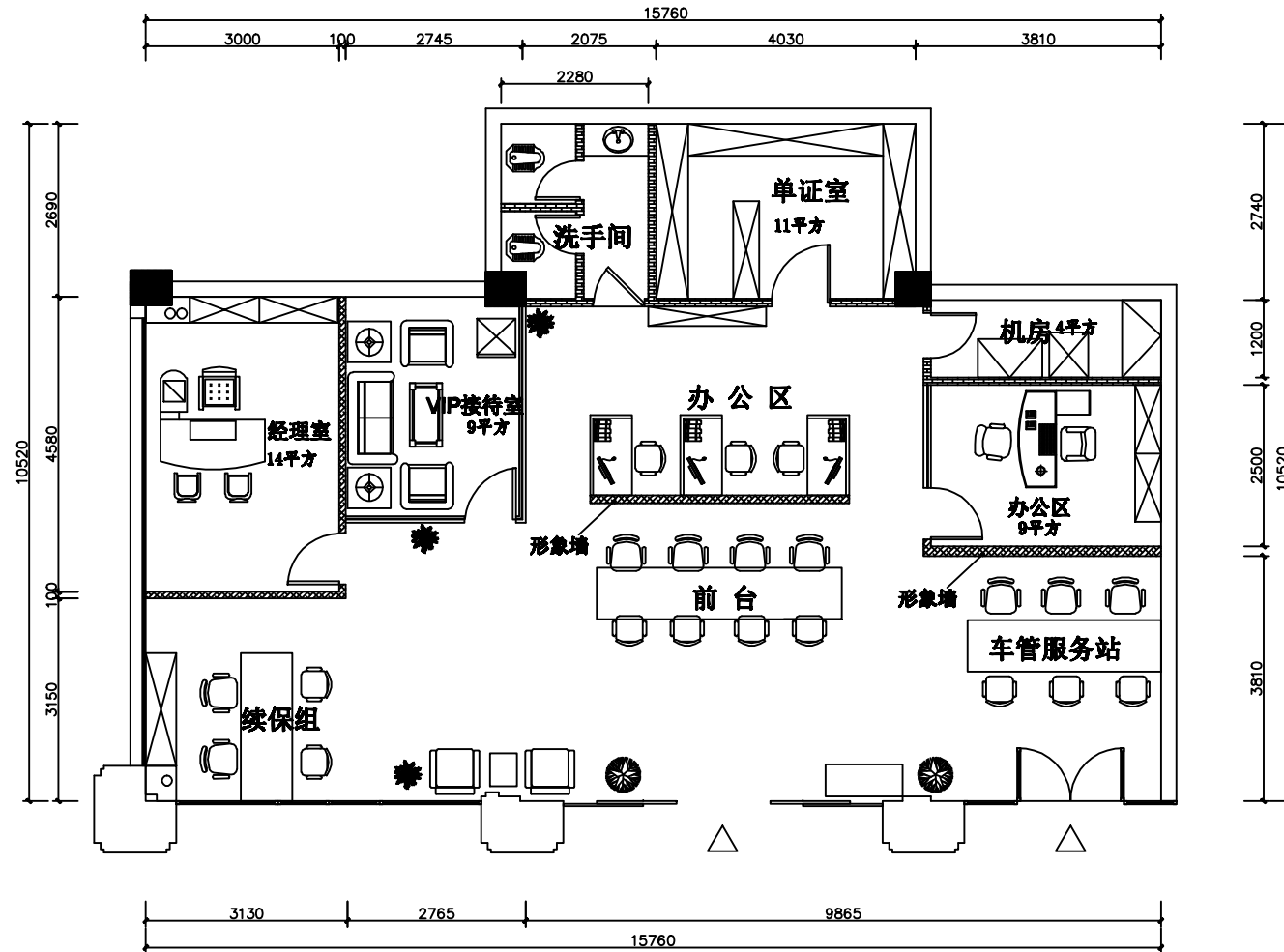
平面布置图1:100
